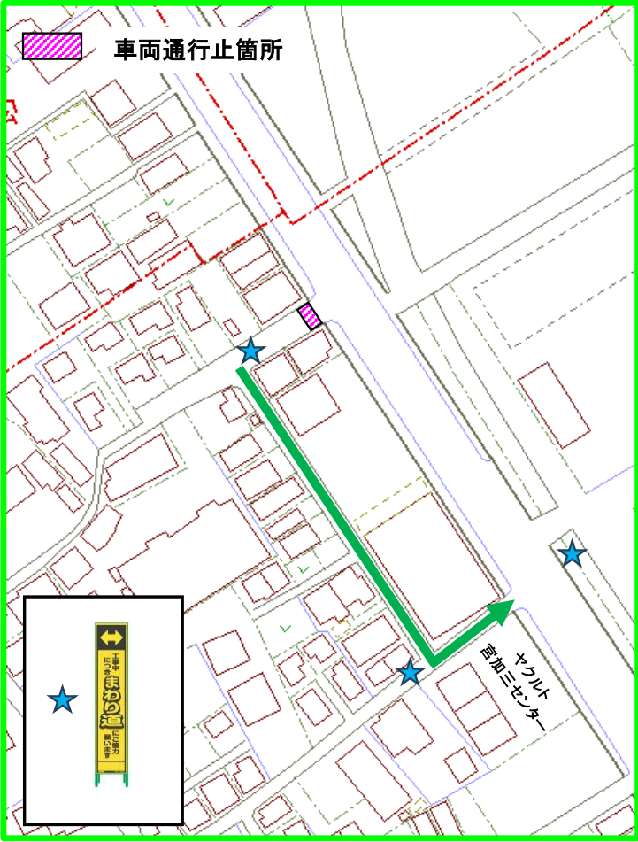
迂回路図【③・⑦施工日】
